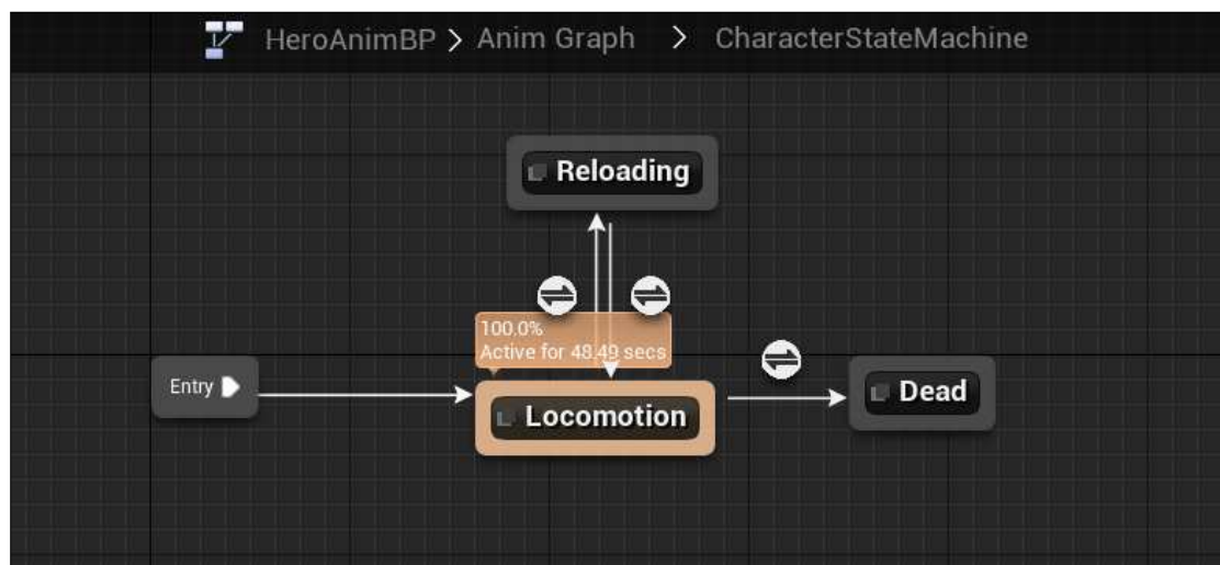
(a) Animační Blueprint postavy a jeho stavový automat.
